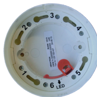
Abb. 6: Der Magnet muss auf Klemme 5 im Sockel eingesetzt werden. Dadurch werden die im Rauchschalter integrierten Abschlusswiderstände über Reedkontakte aktiviert. Wird der Magnet nicht eingesetzt, hat der Rauchschalter wie gewohnt seinen potentialfreien Öffner.
