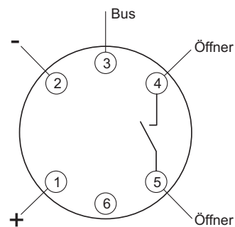
Abb. 4: Interne Beschaltung des ORS 142 bei nicht eingesetztem Magnet
