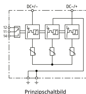
Prinzipschaltbild
