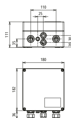
Maßbild
