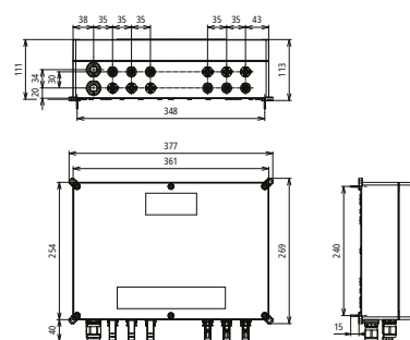
Maßbild
