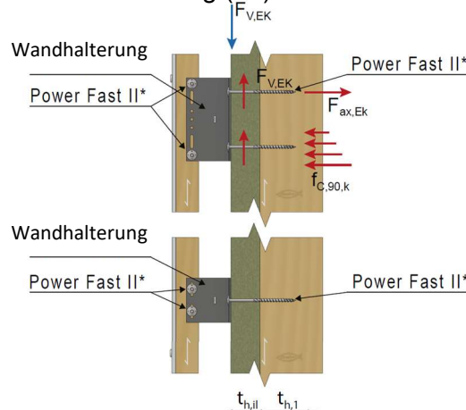
Abbildung F4.1: Anwendung von fischer PowerFast II Schrauben für Systeme mit verschieblichen Zwischenschichten (Abbildung nicht maßstäblich)
