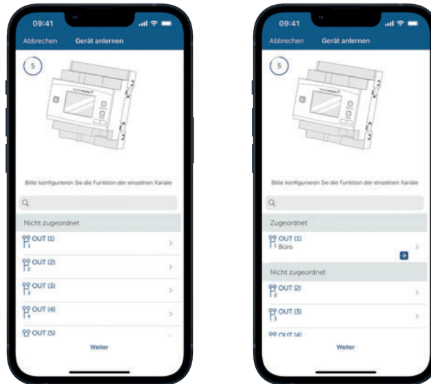
Abbildung 96: Screenshot Kanalkonfiguration bei Ersteinrichtung
