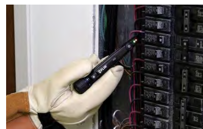
FLIR VP42 helpt bij problemen met werkende en neutrale bedrading en zorgt voor een veilige werksituatie
