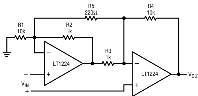
LT1224 • TA09
