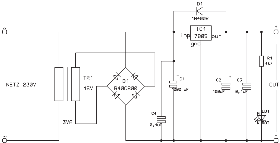
Schaltplan 190822
