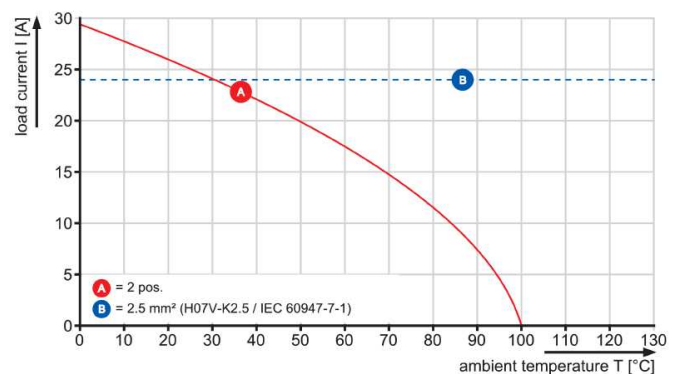
TOP 4GS../180-6.35
