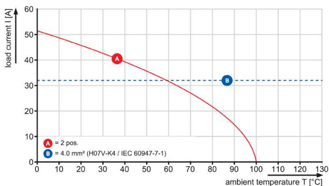
TOP 4GS../90-6.35
