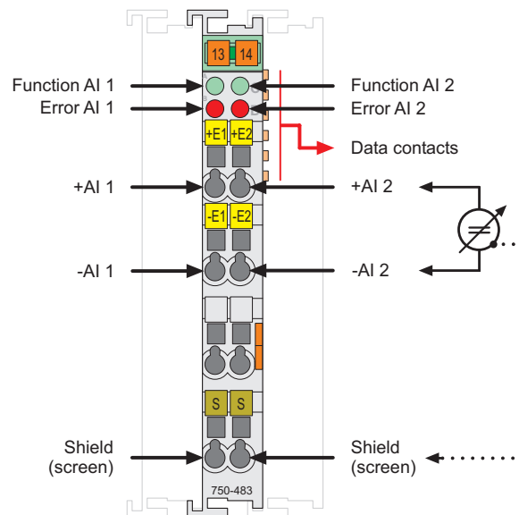
Fig. 2.1.1-1: 2-Channel Analog Input Module DC 0-30 V
