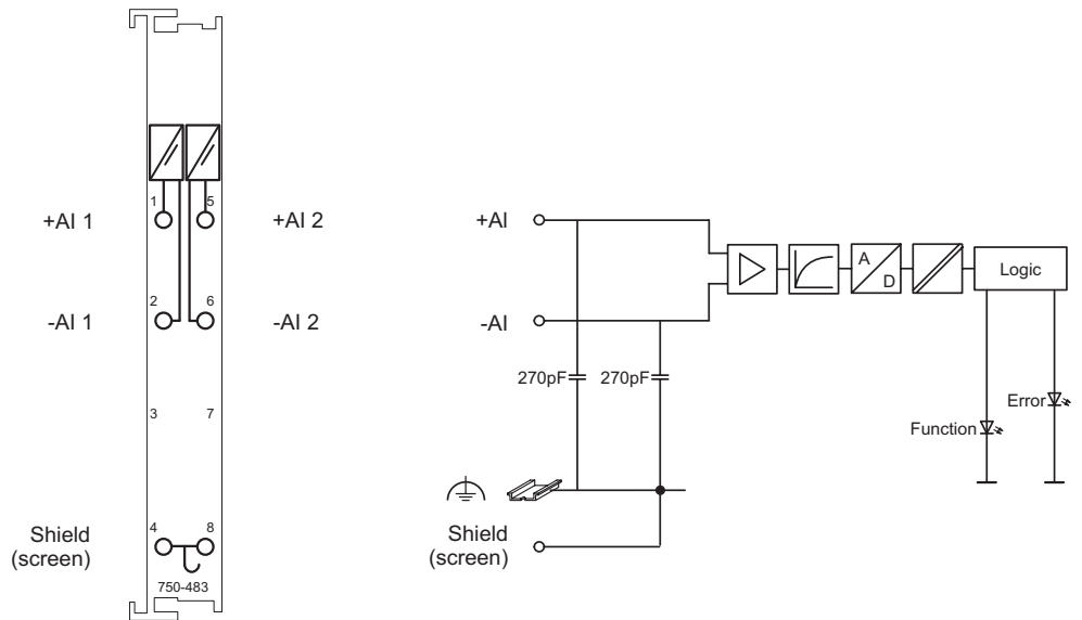
Fig. 2.1.1-3: 2-Channel Analog Input Module 0-30 V
