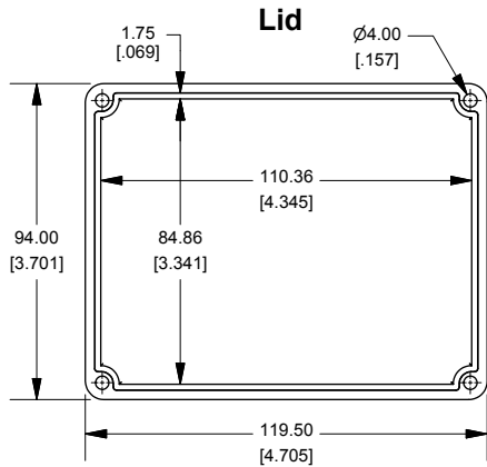
Lid
