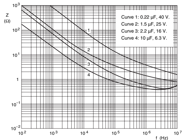
Case size H × W × T = 10 × 7 × 3.5 mm. T amb = 25 °C.
