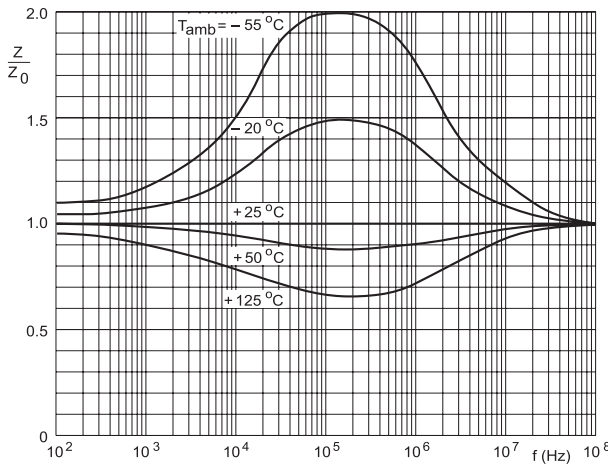
Z 0 = initial impedance value at T amb = 25 °C.
