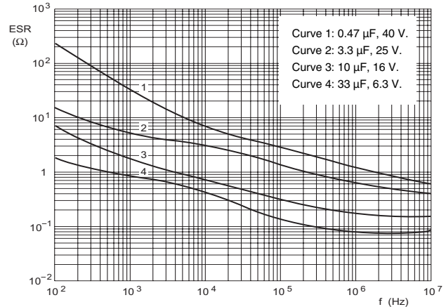
Case size H × W × T = 10 × 7 × 5 mm. T amb = 25 °C.
