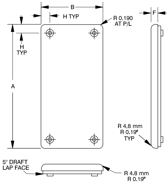
Lid View
