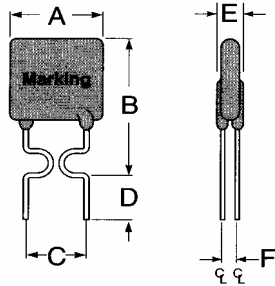
FRU 090-30F ~ FRU 250-30F Lead Size: 24AWG \Phi 0.51 mm Diameter
