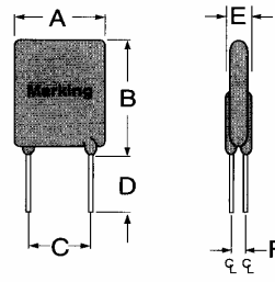
FRU 300-30F ~ FRU 900-30F Lead Size: 20AWG \Phi 0.81 mm Diameter
