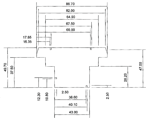
CMEB max pcb dimensions
