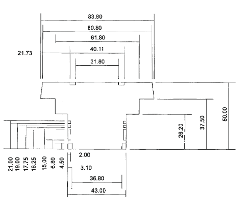
CMEB/E max pcb dimensions
