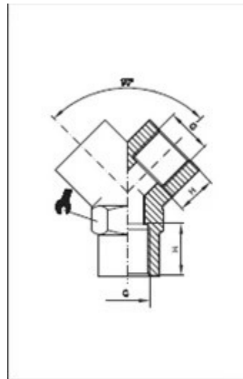
Y-Verteiler Female Y-connector
