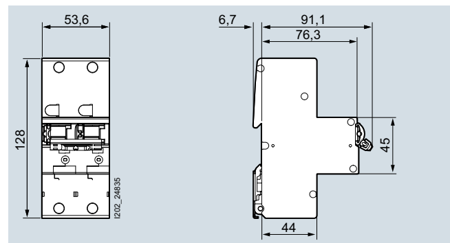
5SP32...-3 2P
