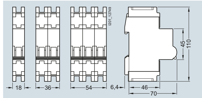
5SJ4...-HG41
