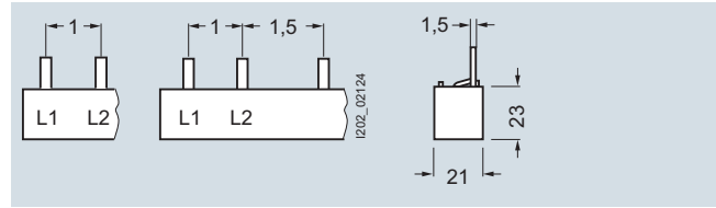
5ST3705-0HG 5ST3707-0HG
