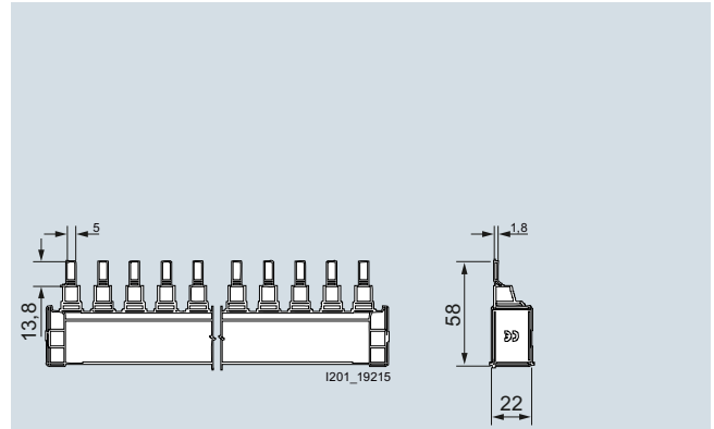
5ST37...-3HG
