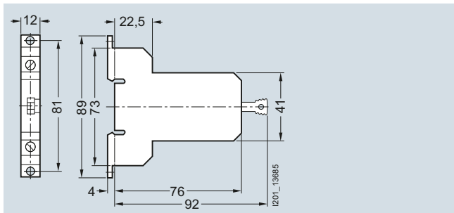
5SK9011-1KK2. 5SK9011-2KK2.
