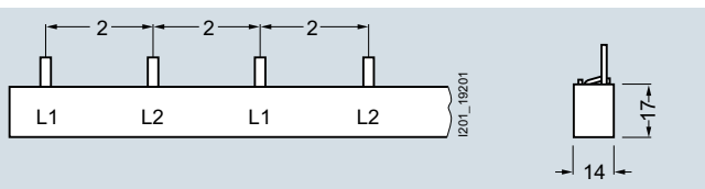
5ST3735-2
