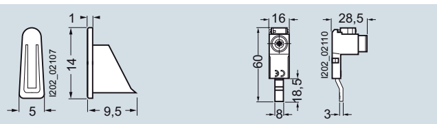
5ST3748-0HG 5ST3770-0HG
