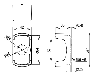
HW9Z-KG3
