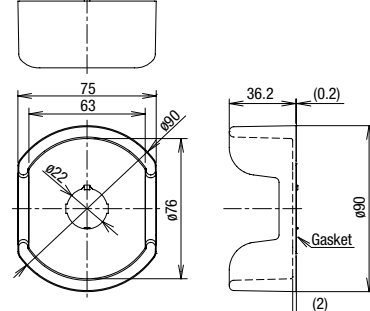
HW9Z-KG5
