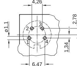
4 POL*
