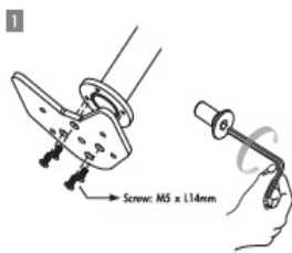
Combine Iron Pipe with Grommet base 組合鐵管與Grommet底座
