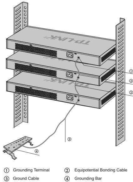
Figure 3-3 Equipotential Bonding
