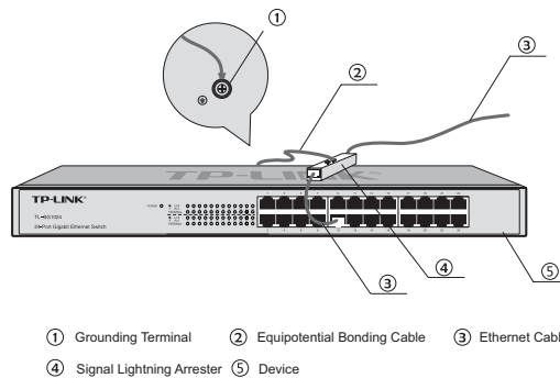
Figure 3-4 Equipotential Bonding
