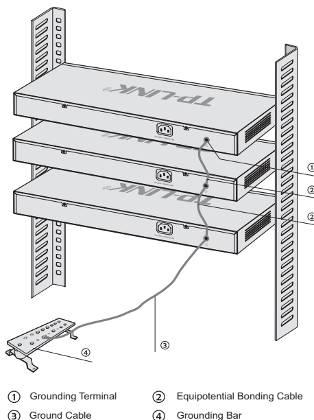
Figure 3-3 Equipotential Bonding
