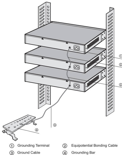
Figure 3-3 Equipotential Bonding
