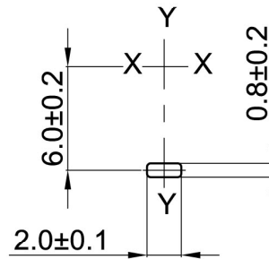
LOCATING LUG DETAIL
