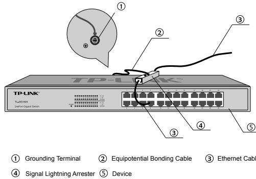
Figure 3-4 Equipotential Bonding
