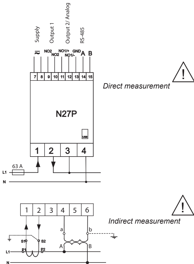
Rysunek 3. Podłączenie elektryczne miernika N27P.
