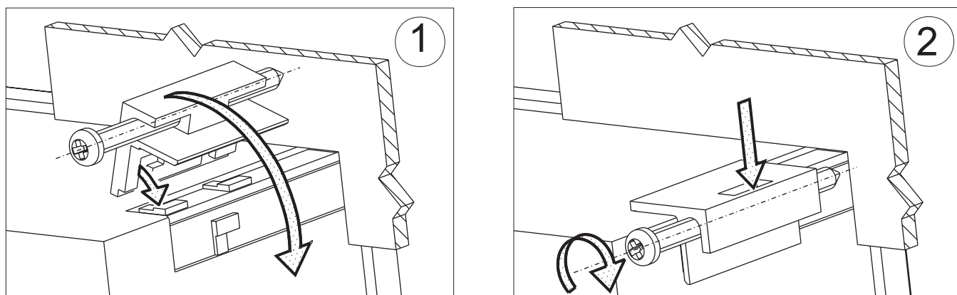
Fig. 2. Meter Fixing
