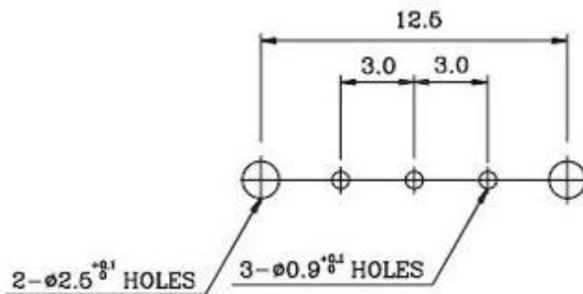
P.C.B LAY OUT
