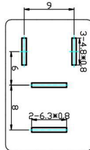
4290 Schematic II
