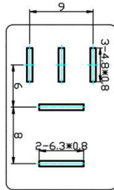
4290 Schematic Z
