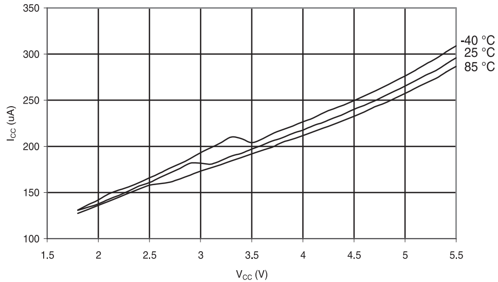
Figure 30-275. ATmega168PA: ADC Current vs. V CC (AREF = AV CC )
