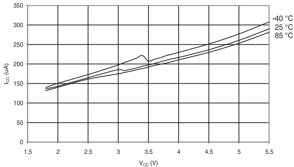
Figure 30-87. ATmega48PA: ADC Current vs. V CC (AREF = AV CC )
