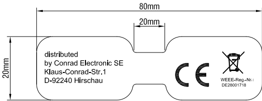
Wire sticker(REV.3)
