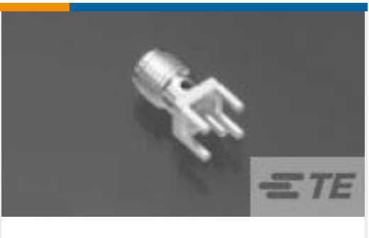
TE Part #1053354-1 2062 0000 00,SMA PCB VERT JACK
