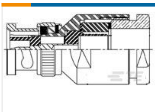
TE Part #1-1478408-0 BNC Str Plg PS 75Ohm Silver URM70
