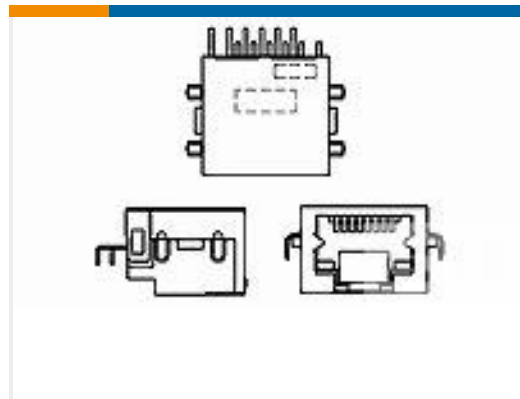
TE Part #3-1734819-5 RJ45 Tab-Down RVS OFST T&R 6u"
