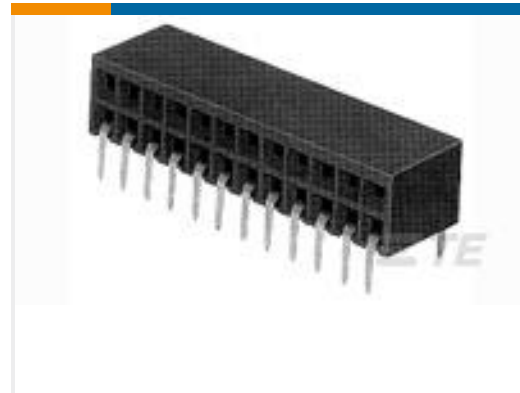
TE Part #6-87961-4 130 MODII HORZ DR CE 100CL/115
