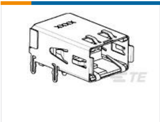
TE Part #1761072-4 RECPT,HSSDC2,FIBRE,ON TAPE
