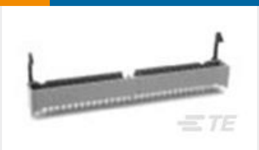
TE Part #2-1761713-5 IDC LOW PRO HDR 14P VERT SHT LAT BLUE
