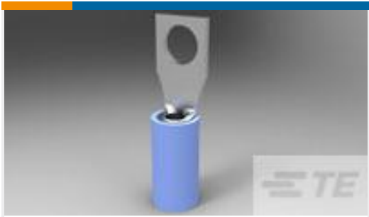
TE Part # 130477 PIDG RECP TONGUE STUD HOLE 4.0
