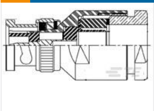
TE Part #1-1478408-0 BNC Str Plg PS 75Ohm Silver URM70
