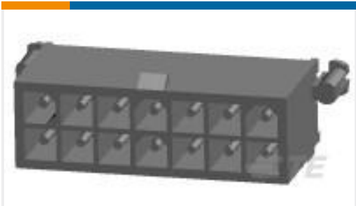
TE Part #1-794074-1 14P MINI UMNL HDR W/O DH AU LF
