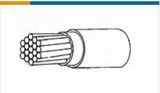
TE Part #218278-000 22759/34-20-90
