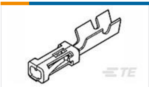
TE Part #1-87523-8 MOD IV RECP PLTD 30 DPLX
