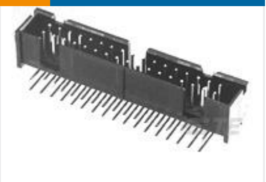
TE Part #103311-6 026 LOPRO HDR RA 30DP
