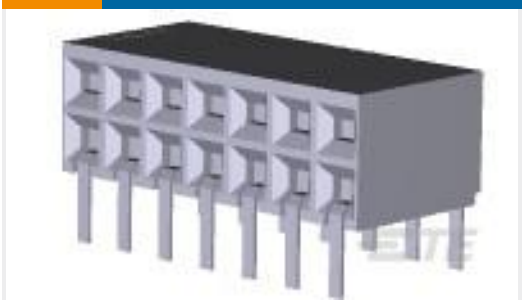
TE Part # 5147722-6 14 MODII HORZ DR SFMNT 30AU
