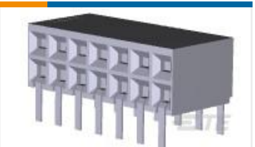
TE Part # 1-147721-3 14 MODII HORZ SR SFMNT 30AU
