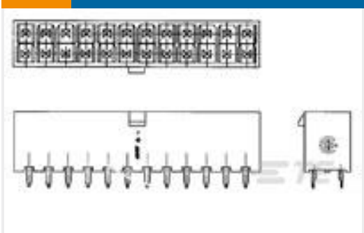
TE Part #1-1586037-6 16P VERT HDR VAL-U-LOK V2
