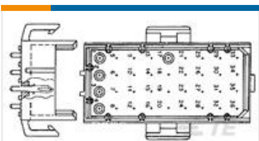
TE Part #2-640503-2 15P MR HDR ASSY VO RED LF
