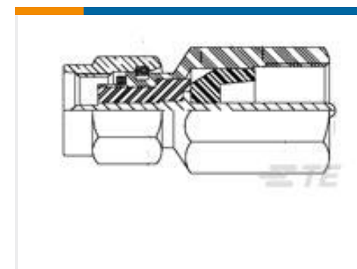
TE Part #1-1337562-0 FME Str Plg-BNCP Adp Nickel Pltd
